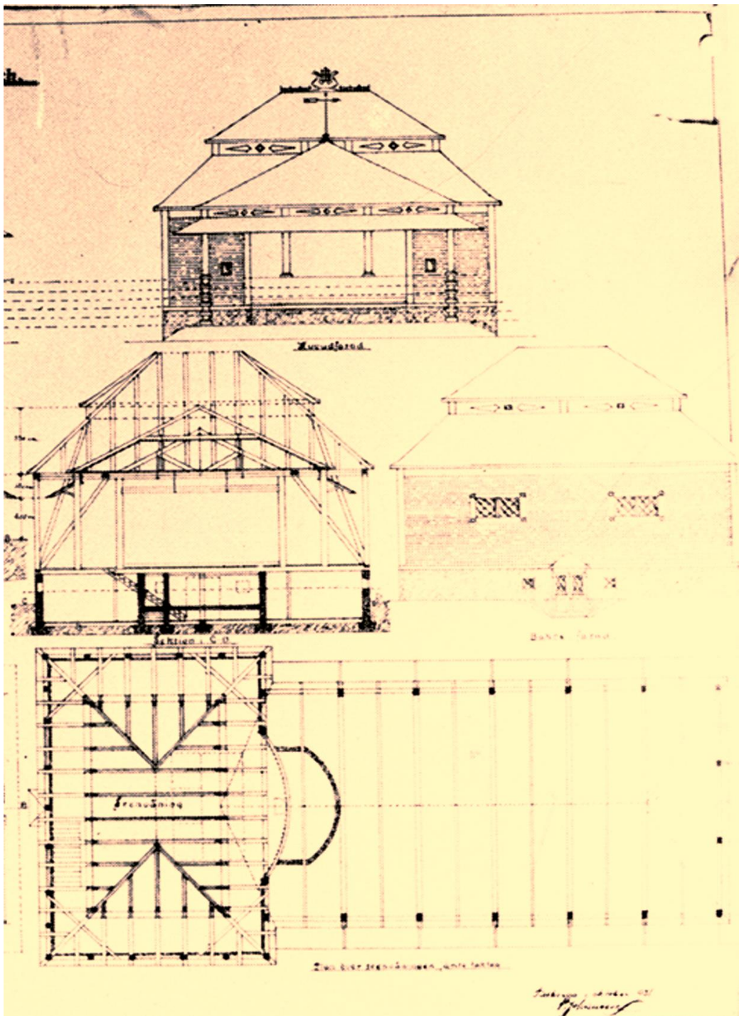
Förslag till teaterbyggnad i Kolbäcks Folkets Park. Ritning från 1931 av byggmästare A. Johansson i Tillberga. (Ritningen är beskuren). Bild: Västmanlands läns museum
